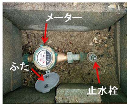
②水道メーターボックス内部
